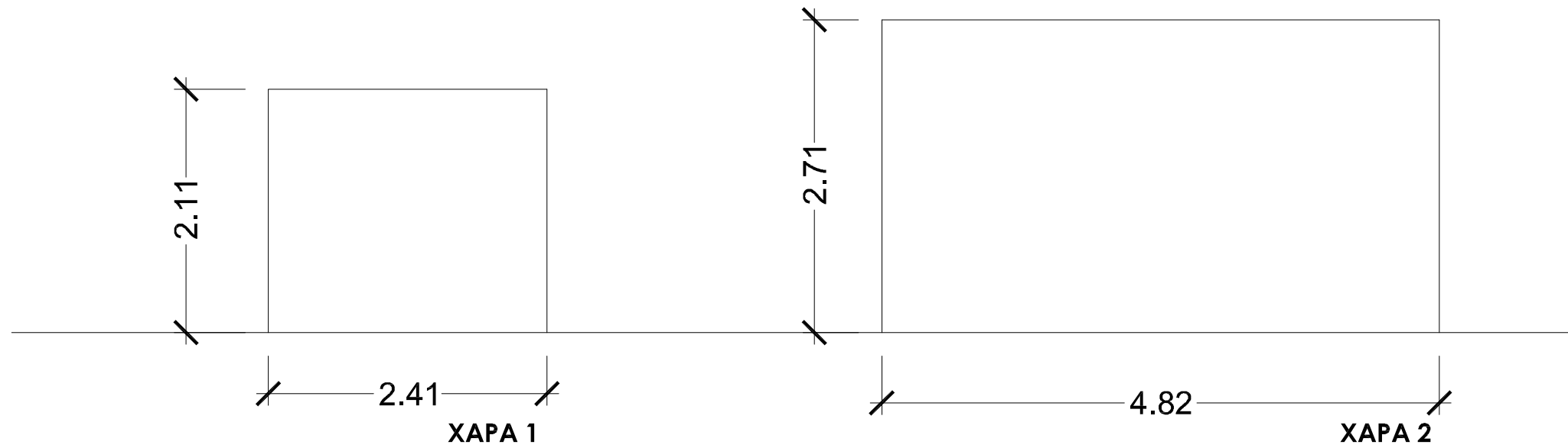
MURS TANCA TRIANGLES Material : Xapa cortén
